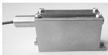
图 5 光纤光栅加速度传感器实物图
