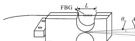
图 1 柔性铰链结构的加速度传感器结构示意图
