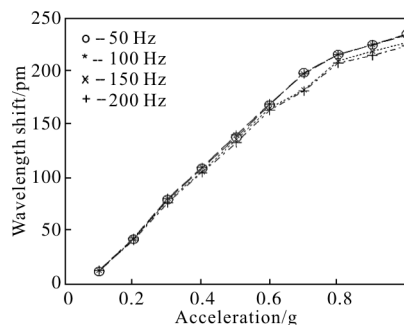
图 10 系统加速度响应曲线
