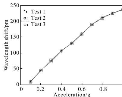
图 11 系统加速度响应重复性曲线
