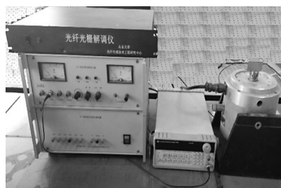
图 7 光纤光栅加速度检测系统性能指标测试平台
