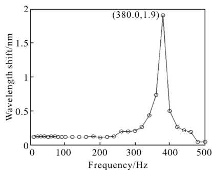
图 9 系统幅频特性曲线
