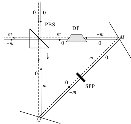
(b) 插入道威棱镜
