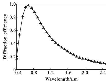
图 2 闪耀角为 1°时光栅衍射效率曲线
