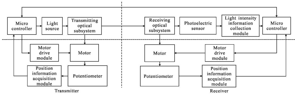
图 5 系统硬件结构图
