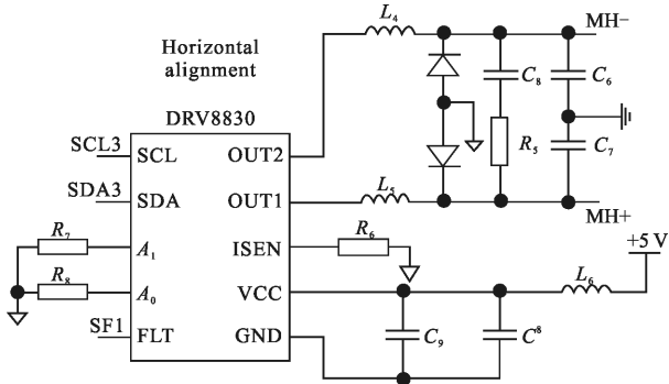
图 7 电机驱动模块电路
