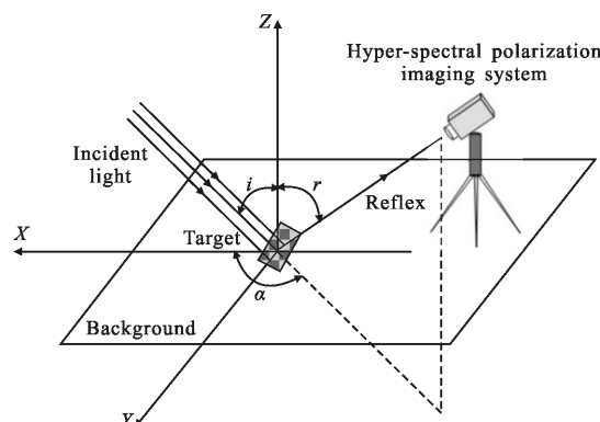
图 5 实验原理图
