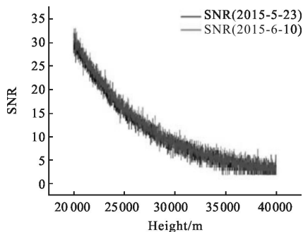
图 5 20~40 km 高度范围激光回波信噪比廓线 Fig.5 Profile of SNR of lidar for height of 20~40 km
