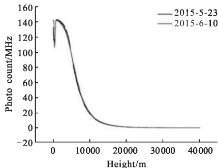
图 3 激光雷达回波信号 Fig.3 Echo signal of lidar
