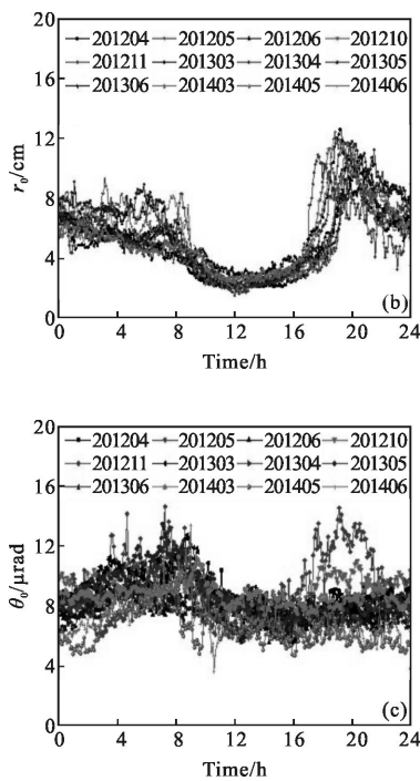
图 3 C_n^2 , r_0 和 \theta_0 月平均值日变化
