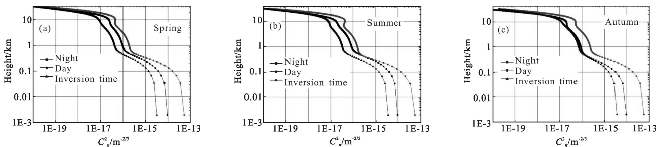
图 6 折射率结构常数拟合模式
