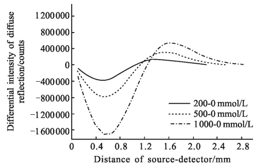
(b) 三种不同浓度 10% intralipid-葡萄糖溶液检测部分光程漫反射光强度差分分布
