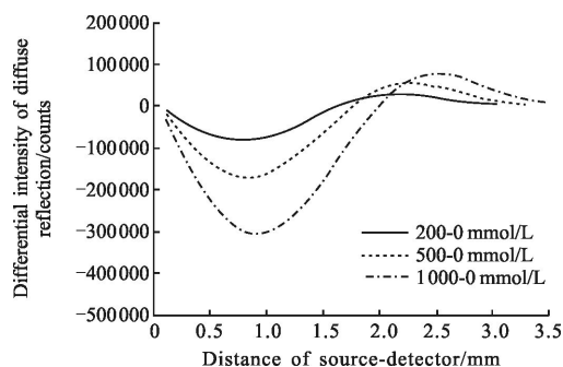
(b) 不同浓度 3% intralipid-葡萄糖溶液检测部分光程漫反射光差分强度分布
