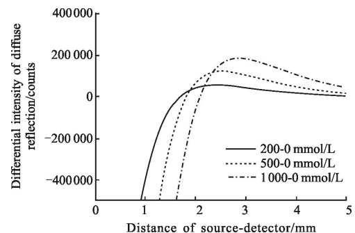
(a) 不同浓度 3% intralipid-葡萄糖溶液全部光程漫反射光差分强度分布
