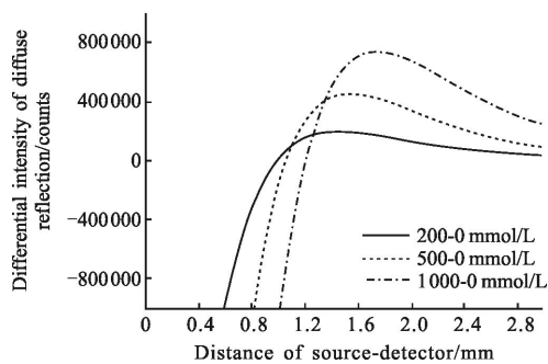
(a) 三种不同浓度 10% intralipid-葡萄糖溶液全部光程漫反射光强度差分分布
