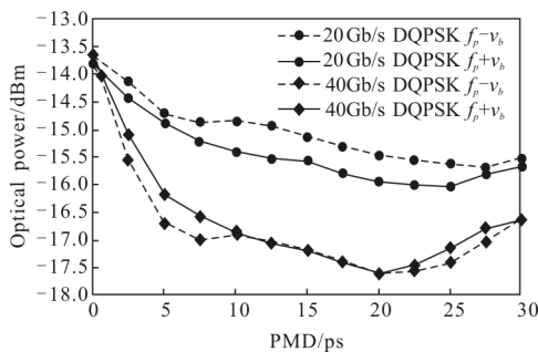
图 3 TOF 中心频率分别为 f_p - v_b 和 f_p + v_b 时的光功率值随 PMD 值的变化
