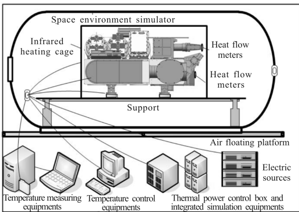
(a) 热平衡实验装置图
