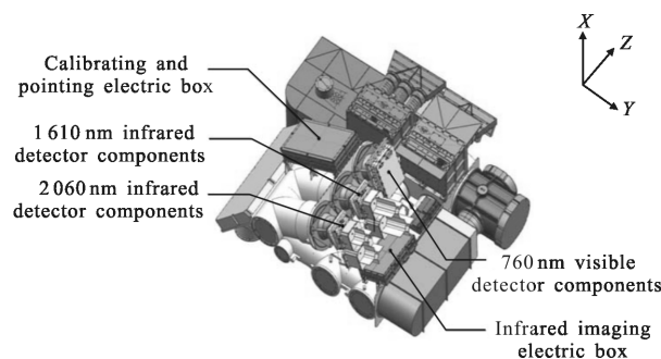
图 1 红外探测器组件位置及探测仪坐标系定义
