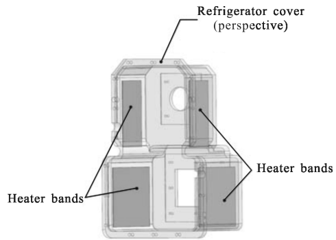
图 5 红外探测器组件加热片布置
