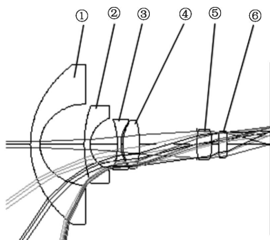
图 2 专利 JP47-42169 的结构图
