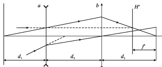
图 1 反远物镜光路图
