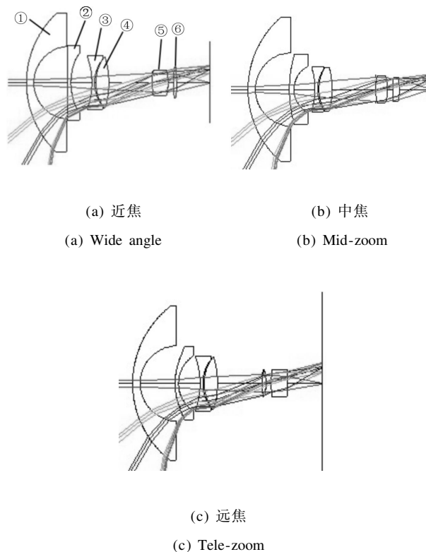
图 3 鱼眼镜头光线追迹图
