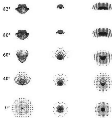
图 4 点列图
