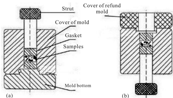
图 1 压片模具组装(a)及退模(b)示意图
