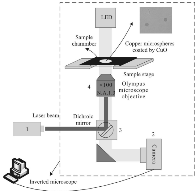
图 5 光镊装置
