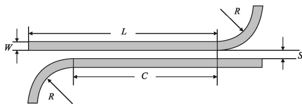
图 2 俯视图
