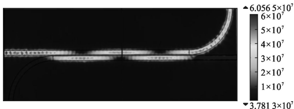
图 4 1.55 μm 波 TE 模通过时波导芯层中心截面上的电场模分布 Fig.4 TE electric field distribution on the waveguide core center of the section at 1.55 μm wavelength
