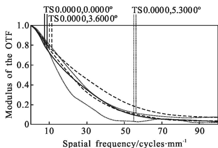
(a) 初始 MTF
