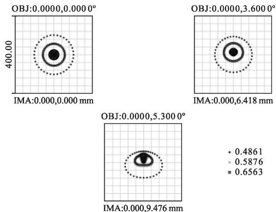
(a) 初始点列图
