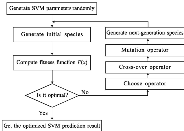
图 4 GA 优化 SVM 流程图
