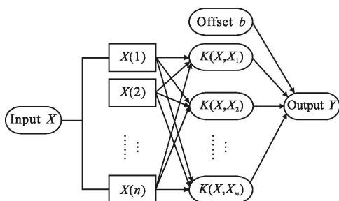
图 1 支持向量机的结构
