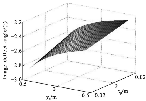
(b) 侧摆 38°焦面偏流角分布
