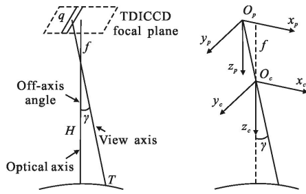
图 2 离轴三反空间相机简化模型
