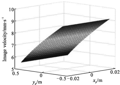
(a) 侧摆 38°焦面像移速度分布
