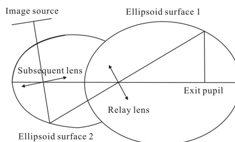
图 1 双椭球结构系统示意图
