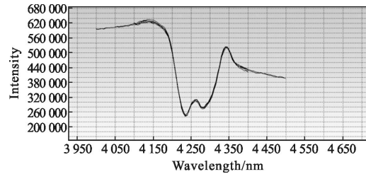
图 7 4.0~4.5 μm 通氮气整体光谱曲线
