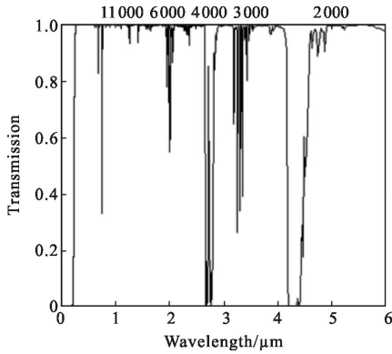
图 4 地面 CO 2 透过率曲线
