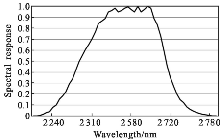
图 9 红外通道整机光谱响应曲线
