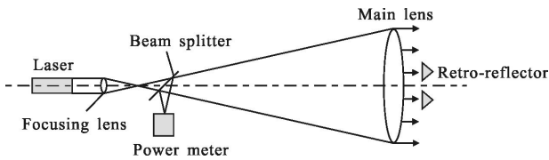
图 3 有效反射面积测试原理图
