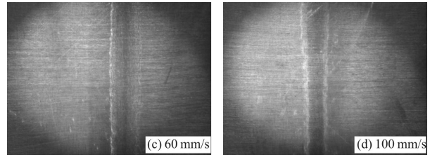
图 5 焊接速度对焊缝显微组织的影响(激光功率为 40 W,透明塑料厚度为 3 mm,放大倍数为 20 X)
