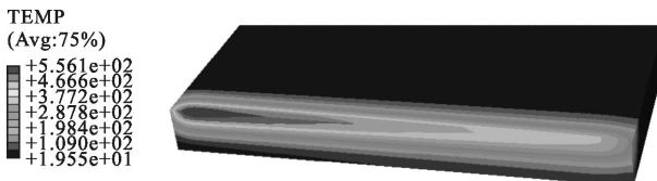
(b) 焊接速度为 20 mm/s (b) Welding speed=20 mm/s
