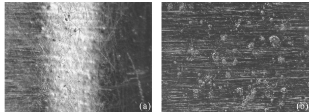
图 7 焊接区域的显微组织(放大倍数 200 X)
