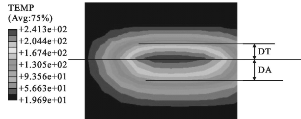
图 3 焊接数值模拟中获得透明和吸收 PC 塑料的熔融深度
