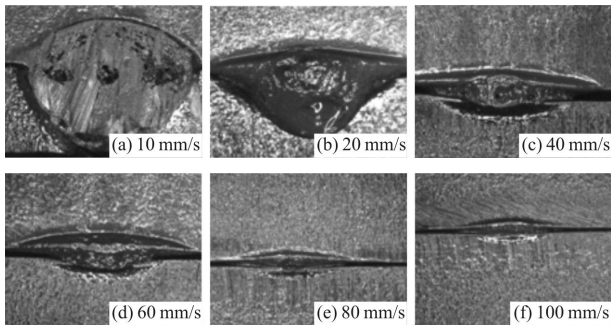
图 4 焊接实验中获得透明和吸收 PC 塑料的熔融深度 (放大倍数为 50 X)
