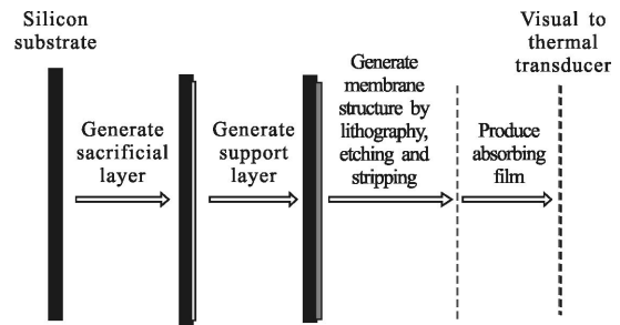
图 2 转换膜的制作流程
