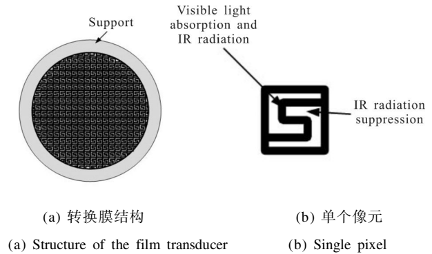
图 1 可见光/红外图像转换的膜结构示意图
