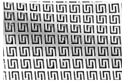
图 4 显微镜下的转换膜结构
