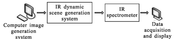
图 5 红外光谱范围测试实验装置原理框图
