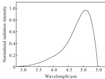
(a) 3~5 μm 红外窗口
