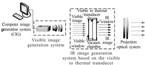
图 3 红外动态图像生成装置组成
