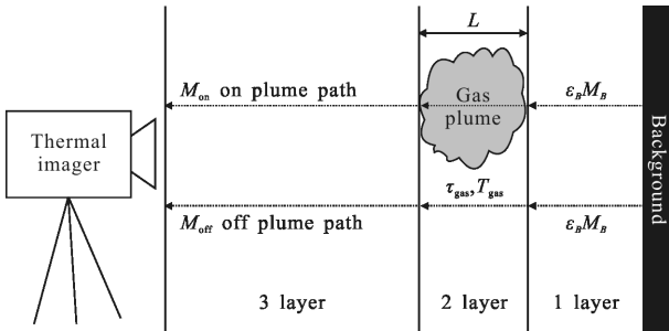
图 1 3 层辐射传输模型示意图
