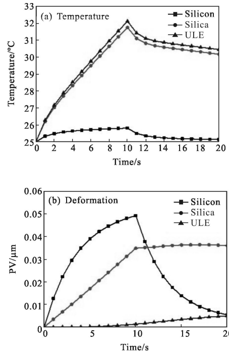
图 4 由单晶硅、石英与 ULE 制作的变形镜在连续激光辐照 10 \text{ s} 后的温升与最大变形分布结果
