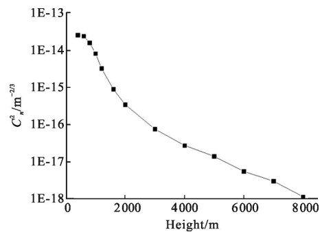
图 5 2015 年 5 月南京实验测得的 C_n^2 廓线 Fig.5 C_n^2 profile for Nanjing, May 2015
