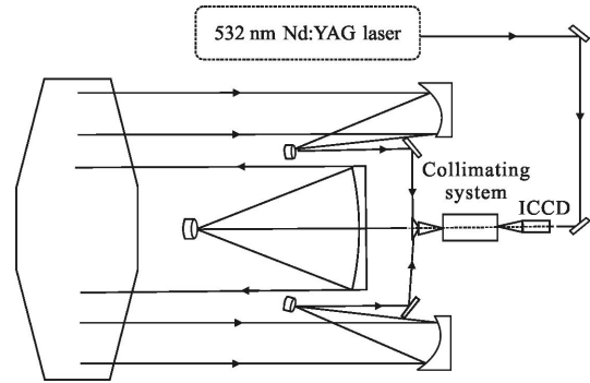
图 1 DIM 激光雷达光路系统图
