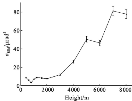
图 4 2015 年 5 月南京实验测得大气差分像移数据 Fig.4 Averaged DIM for image data collected in Nanjing on May, 2015
