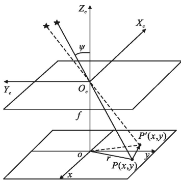
图 2 星敏感器的旋转运动 Fig.2 Rotation of the star tracker
