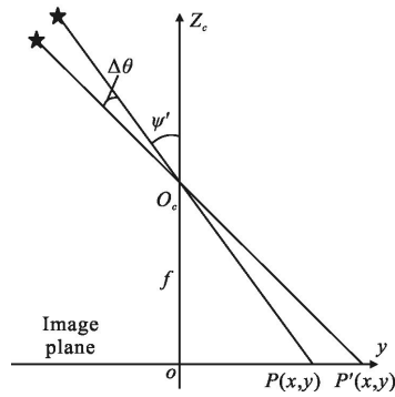
图 3 星敏感器绕 X_c 轴转动 \Delta\theta 角度 Fig.3 Star tracker rotating \Delta\theta around X_c axis
