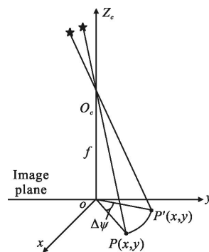
图 4 星敏感器绕 Z_c 轴转动 \Delta\psi 角度 Fig.4 Star tracker rotating \Delta\psi around Z_c axis
