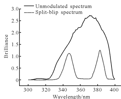
图 2 光源光谱调制曲线图
