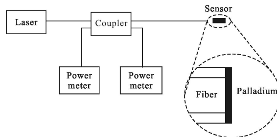
图 1 微透镜型光纤氢气传感系统的光路结构
