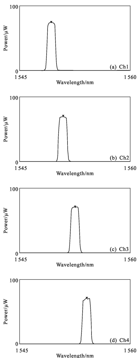
图 6 DWDM1 输出信号的光谱
