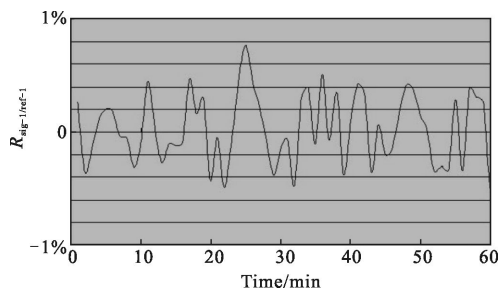
图 10 1 小时内信号光功率和参考光功率的实时比值与平均比值的差异
