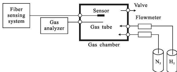
图 3 光纤氢气传感实验装置
