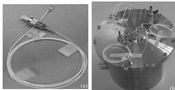
图 4 光纤氢气传感头和测试气室
