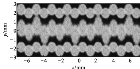
图 9 内环集束入射角度调整后,所有集束在腔壁的光斑叠加
