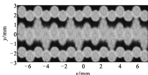
图 8 内环集束焦面位置调整后,所有集束在腔壁的光斑叠加
