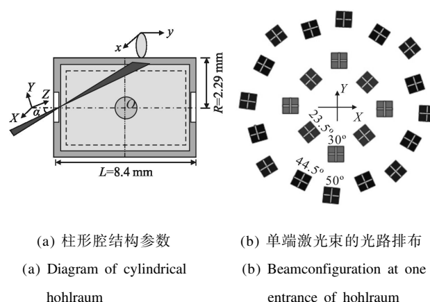
图 1 柱形腔结构示意图
