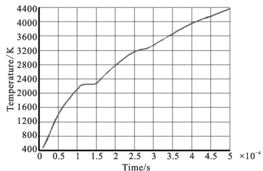
图 7 脉冲激光辐照靶材中心点温度变化曲线
