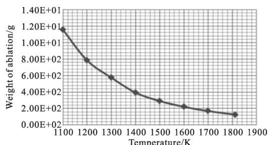
图 10 不同剥离温度点时的剥离质量
