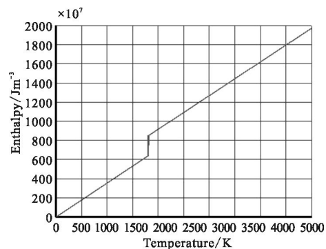
图 2 铁的焓-温度曲线
