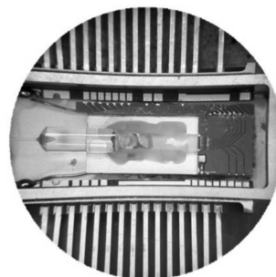
(b) 封装实物图
