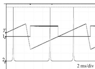
图 2 最大输出功率 140 mW 的单频输出测量
