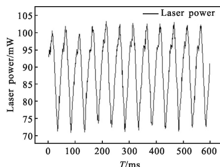
图 6 RTP 晶体周期性加电的线性调频输出功率变化
