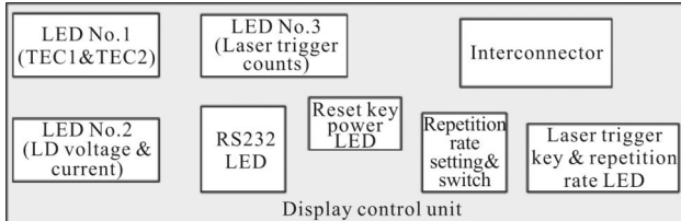
图 4 显示控制组件功能组成框图
