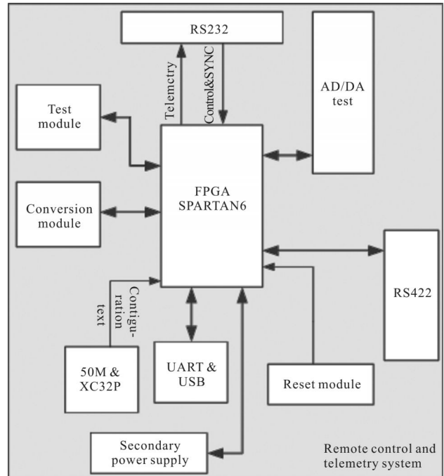
图 3 遥控遥测组件功能组成框图
