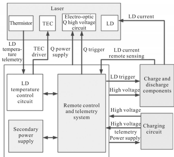
图 1 激光激励电源功能组成示意图
