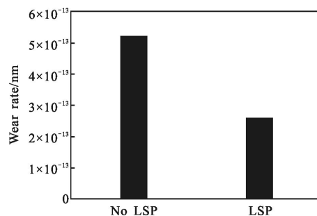
图 1 304 不锈钢激光冲击强化前后的比磨损率图
