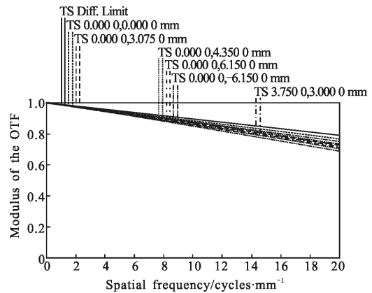
图 3 光学系统 MTF 曲线图
