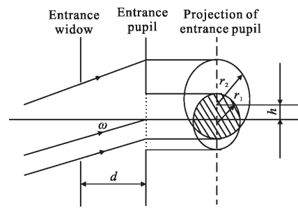
图 1 成像光束光路图
