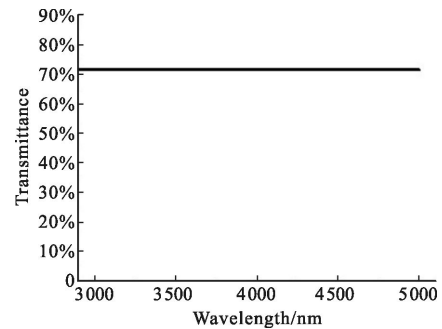
图 1 金刚石在 3~5 \mu\text{m} 波段的透射率曲线
