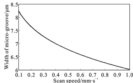
(b) 槽宽
