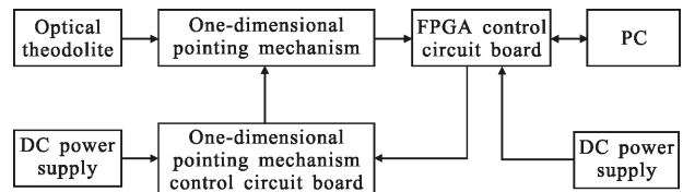
图 9 实验平台系统框图
