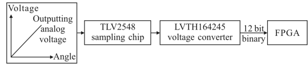
图 8 测角电路示意图
