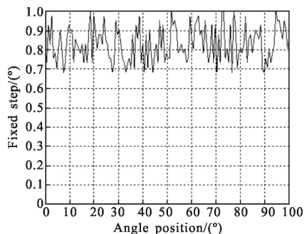
图 12 指向范围内不同位置固定步长
