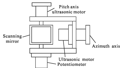
图 2 基于超声电机及电位计的二维指向机构示意图
