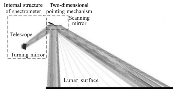
图 1 光谱仪二维目标可选探测工作原理
