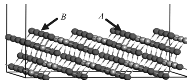
图 1 锐钛矿相 \text{TiO}_2(101) 无氧空位表面原子结构模型
