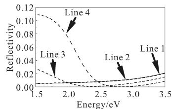
图 6 吸附前后锐钛矿 TiO 2 (101)表面的反射谱
