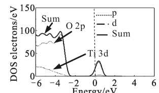
(d) 两个 O 空位表面的态密度 (d) Surface with two oxygen vacancies density of states
