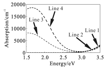
图 5 吸附前后锐钛矿 TiO 2 (101)表面的吸收谱
