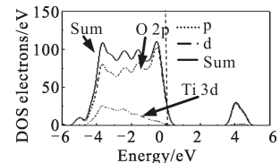
(b) 无 O 空位表面吸附 CO 2 分子后的态密度 (b) Density of states after CO 2 molecules adsorption on anatase TiO 2 (101) surface
