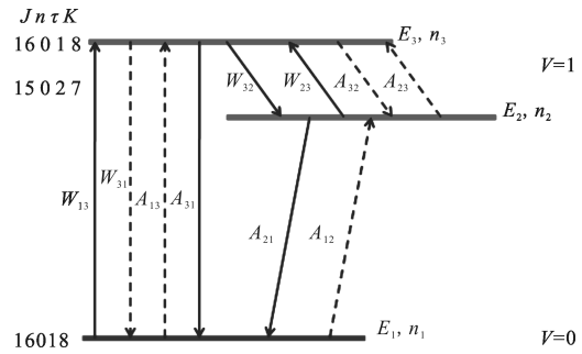
图 1 简化三能级系统模型
