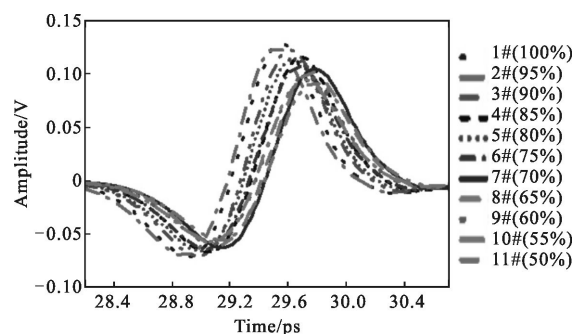
图 1 不同浓度 2,4,4-TMP 与烷基化汽油混合的时域波形 Fig.1 Time-domain spectra of 2,4,4-TMP 1-X AG X (X=50%~100%)
