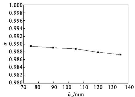
图 10 混合管波瓣瓣高对红外抑制器总压恢复系数影响
