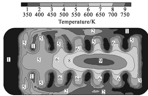
(b) 矩形波瓣出口
