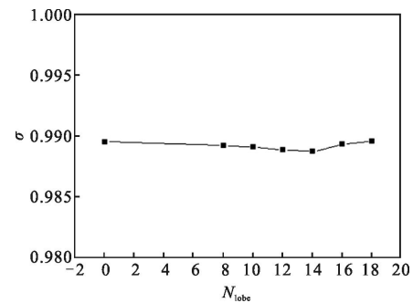
图 9 混合管波瓣数对红外抑制器总压恢复系数影响
