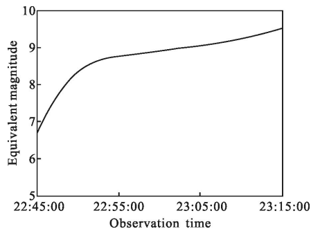
图 4 目标等效星等
