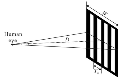
图1 四杆靶图案观测视角示意图
