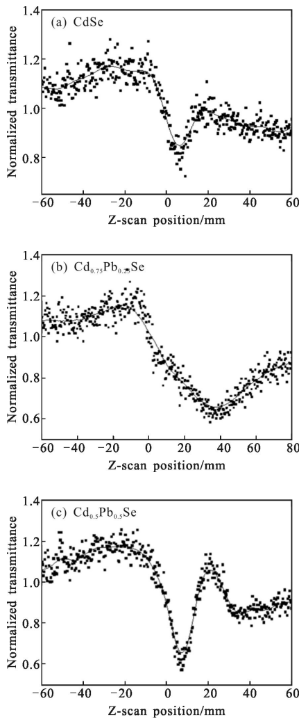
图 4 Cd x Pb 1-x Se 量子点溶液 Z 扫描归一化实验曲线
