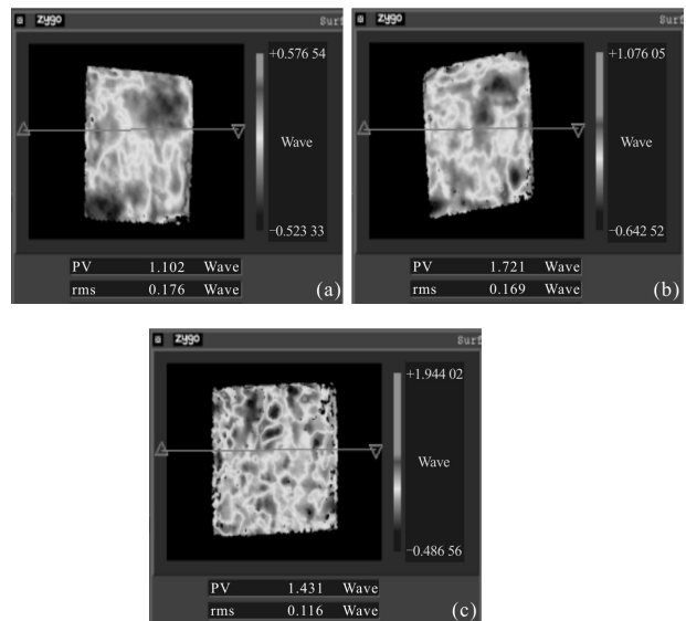
图 9 最终±0.7 视场和 0 视场波面误差等高图
