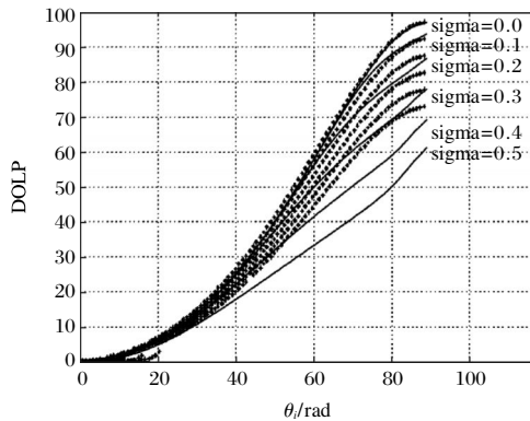
图 5 与 Lawrence 模型仿真对比图 Fig.5 Compare with Lawrence' simulation
