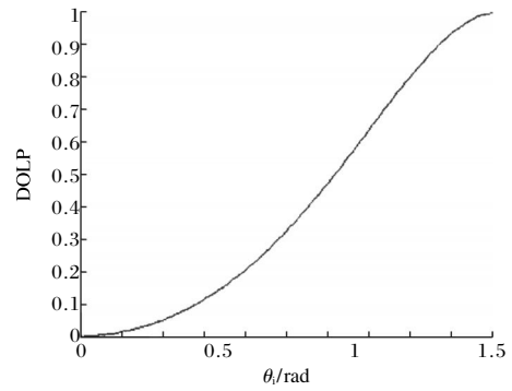
图 3 线偏振度和入射角之间关系(光滑表面)
