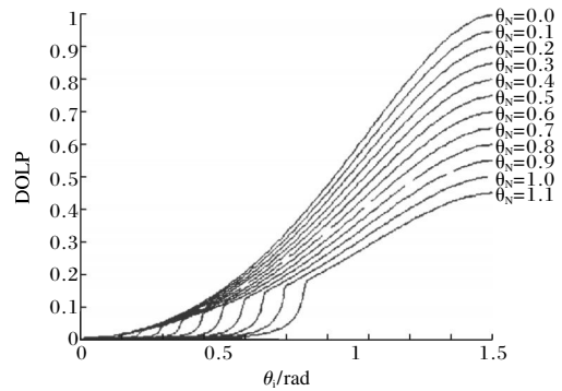
图 4 线偏振度和入射角之间关系(粗糙表面)
