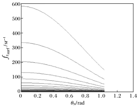
图 2 不同粗糙程度表面 BRDF 值 Fig.2 Value of BRDF in different roughness
