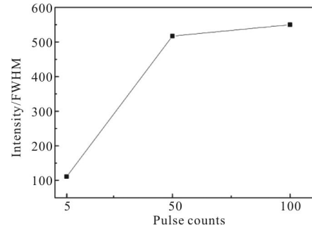
图 5 非晶硅在不同脉冲数下的晶化效果
