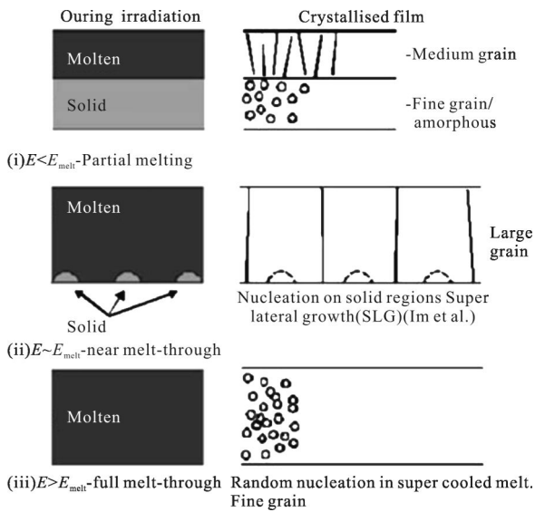
图 6 激光退火过程中 a:Si 熔化阶段示意图以及薄膜中晶粒的组成 [1]
