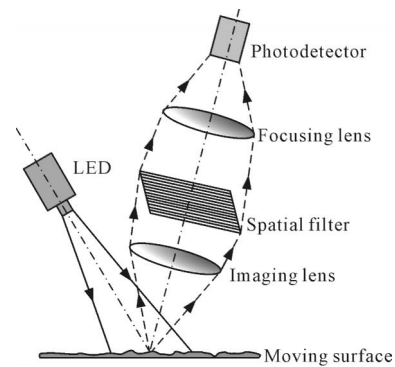
图 1 空间滤波测速仪的基本原理
