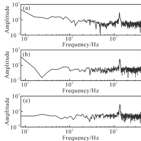
图 7 三种不同结构滤波器典型输出信号的频谱图
