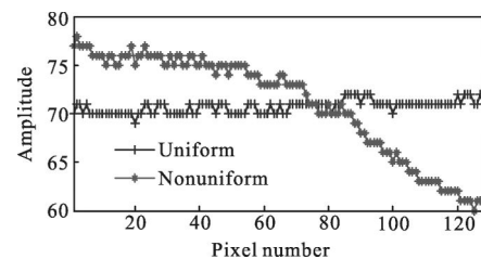
图 4 均匀和非均匀照明下线阵图像传感器的典型输出
