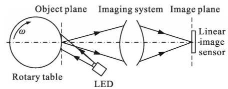
图 3 空间滤波测速仪的实验装置示意图
