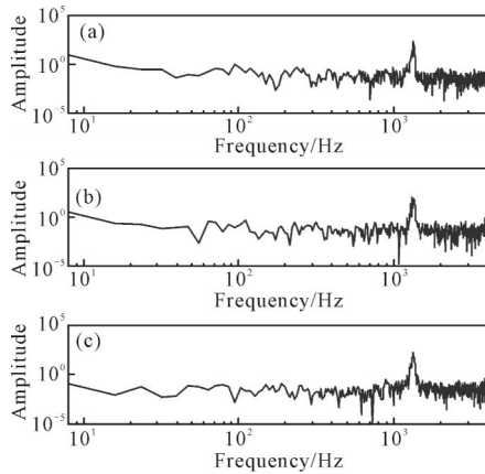
图 5 三种不同结构滤波器典型输出信号的频谱图
